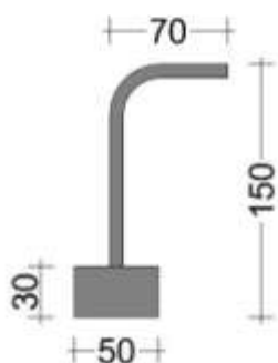
Výztuž Ø 8mm
