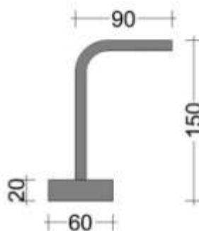
Výztuž Ø 10mm se sníženou výškou boxu
