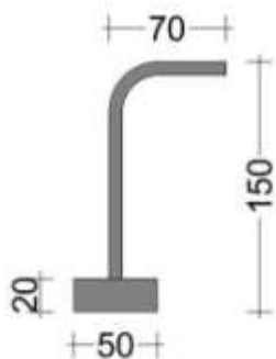
Výztuž Ø 8mm se sníženou výškou boxu
