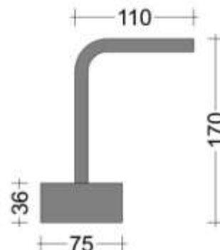
Výztuž Ø 12mm
