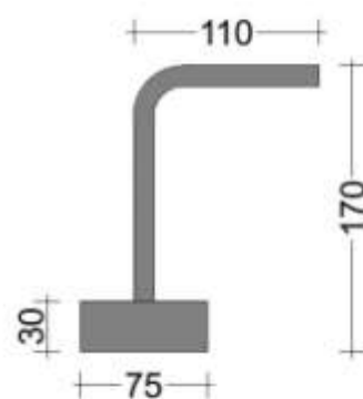
Výztuž Ø 12mm se sníženou výškou boxu
