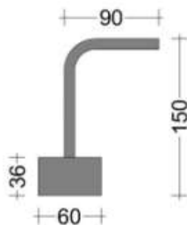
Výztuž Ø 10mm
