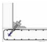
Schéma kotvení V - halter
