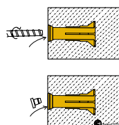
Postup instalace hmoždiny UNI
